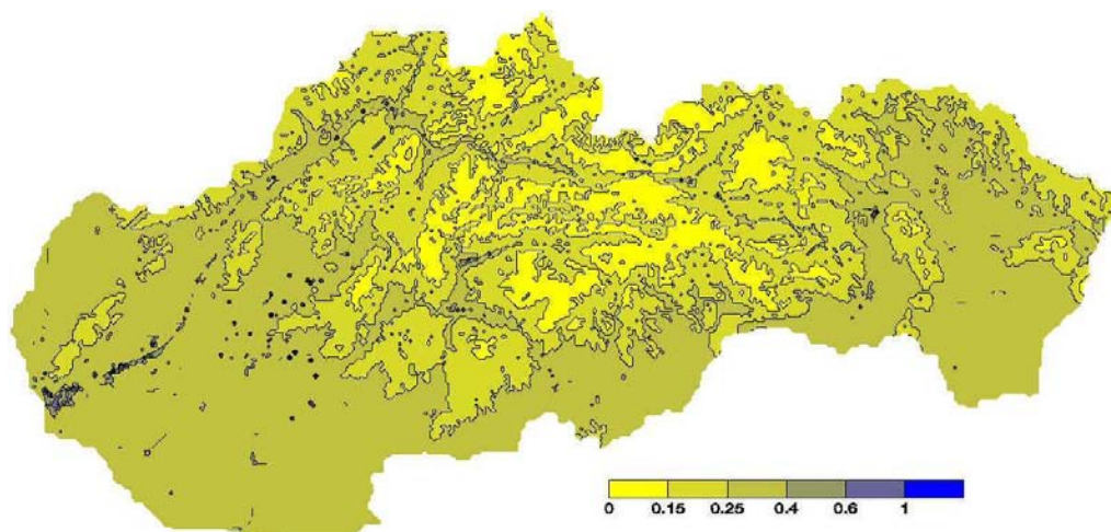
Obr. 5.8 Priemerná ročná koncentrácia benzénu [ \mu\text{g.m}^{-3} ], rok 2013.
