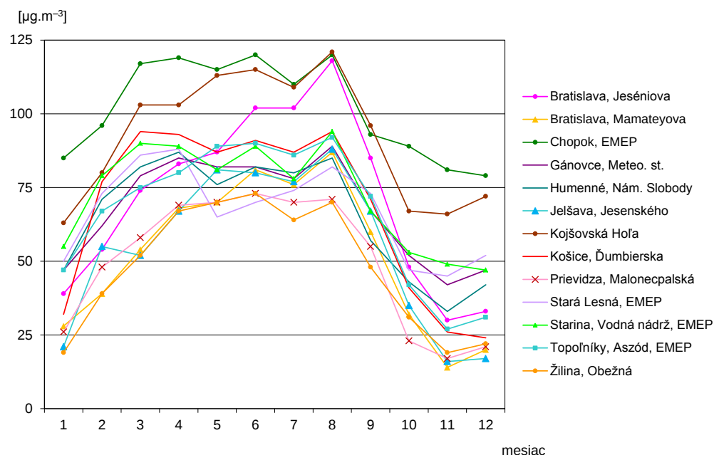
Obr. 4.2 Priemerné mesačné koncentrácie prízemného ozónu na Slovensku v roku 2003.
