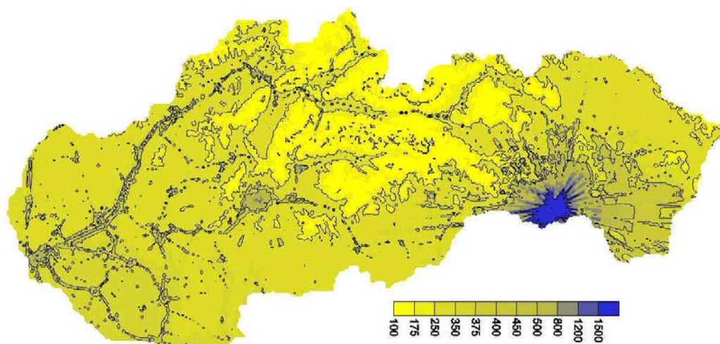
Obr. 5.7 Maximálne denné 8-hodinové kľzavé priemerné koncentrácie [ \mu\text{g.m}^{-3} ] oxidu uhoľnatého (CO), rok 2013.
