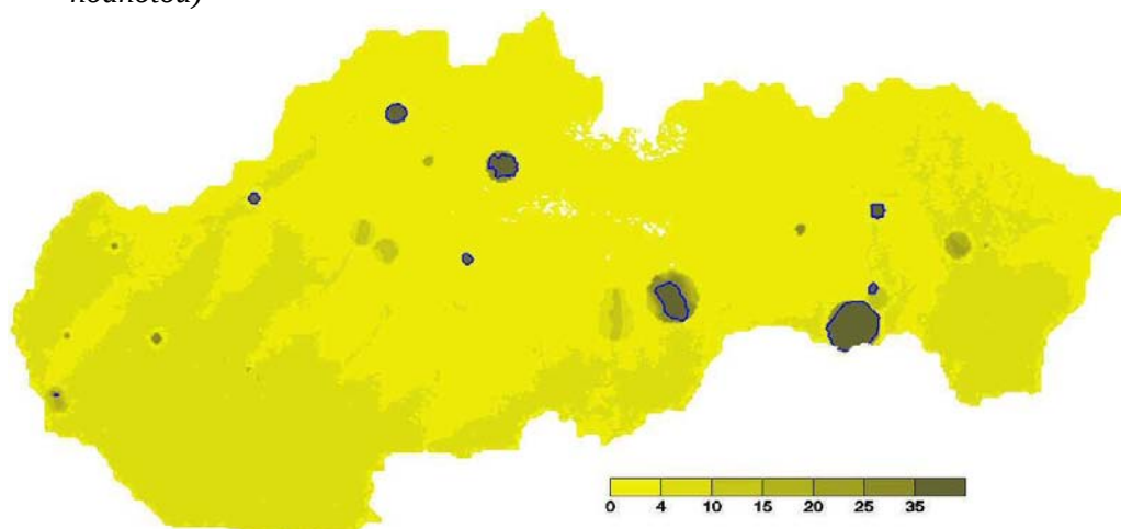
Obr. 5.13 Počet dní s prekročením limitnej hodnoty pre 24-hodinovú koncentráciu PM_{10} ( 50 \mu g \cdot m^{-3} ) v roku 2014. (modrá čiara ohraničuje územie s prekročenou limitnou hodnotou)
