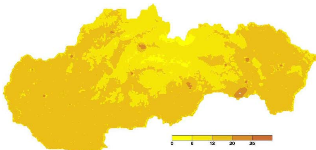
Obr. 5.14 Priemerná ročná koncentrácia PM_{2,5} [ \mu g \cdot m^{-3} ], rok 2014. (modrá čiara ohraničuje územie s prekročenou limitnou hodnotou platnou pre rok 2014, biela čiara je prekročenie cieľovej limitnej hodnoty)
