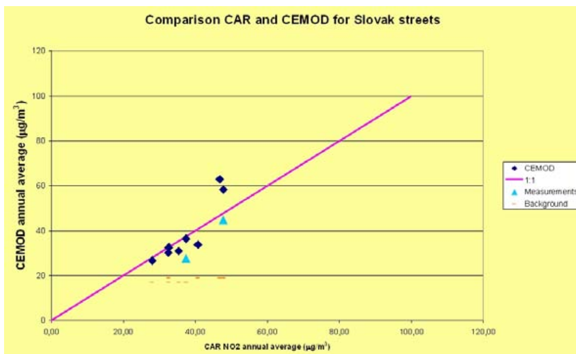
Obr. 4.2 Porovnanie modelov CAR a CEMOD pre \text{NO}_2 .
