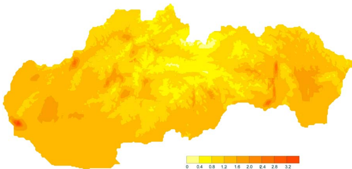
Obr. 4.3 Izočiary priemerných ročných koncentrácií v \mu\text{g.m}^{-3} – benzén rok 2003.
