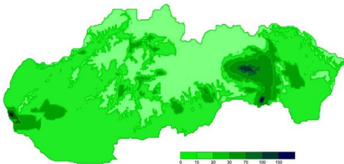
Obr. 4.4 Izočiary priemerných ročných koncentrácií v \mu\text{g.m}^{-3} – olovo rok 2002.
