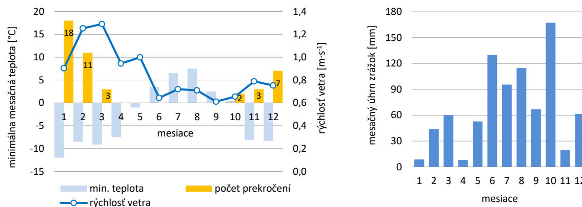
Obr. 3.8 Počet dní s priemernou dennou koncentráciou PM_{10} > 50 \mu g \cdot m^{-3} na AMS Jelšava, Jeséniova v roku 2020 – porovnanie s minimálnou mesačnou teplotou, rýchlosťou vetra a úhrnom zrážok.
