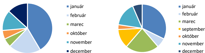
Obr. 3.2 Počet dní s priemernou dennou koncentráciou PM_{10} > 50 \mu g \cdot m^{-3} na aspoň jednej stanici v zóne Banskobystrický kraj (vľavo) a aglomerácii Košice (vpravo) – rozdelenie podľa mesiacov.
