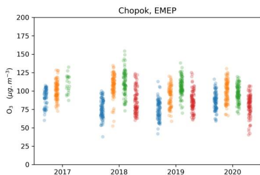
Obr. 3.15 Priemerné denné koncentrácie prízemného ozónu na monitorovacích staniciach Bratislava, Jeséniova; Bratislava, Mamateyova a Chopok, EMEP.
