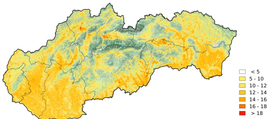
Obr. 4.3 Priemerné ročné koncentrácie PM_{2,5} [ \mu g \cdot m^{-3} ], v roku 2020.
